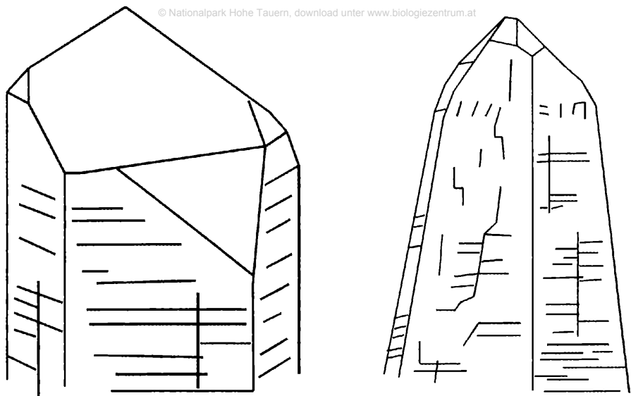
Abb. 1: Quarzkristall mit prismatischem Habitus von Innergschlöß, Venedigergruppe (links), und mit spitzrhomboedrischem Habitus (Tessin-Habitus) vom Hocharn, Großes Fleißtal, Goldberggruppe (rechts) Fig. 1: Quartz crystal with prismatic habit from Innergschlöß, Venediger-group (left), and with acute rhombohedral habit (Tessin habit) from Hocharn, Great Fleißvalley, Goldberg-group (right)
