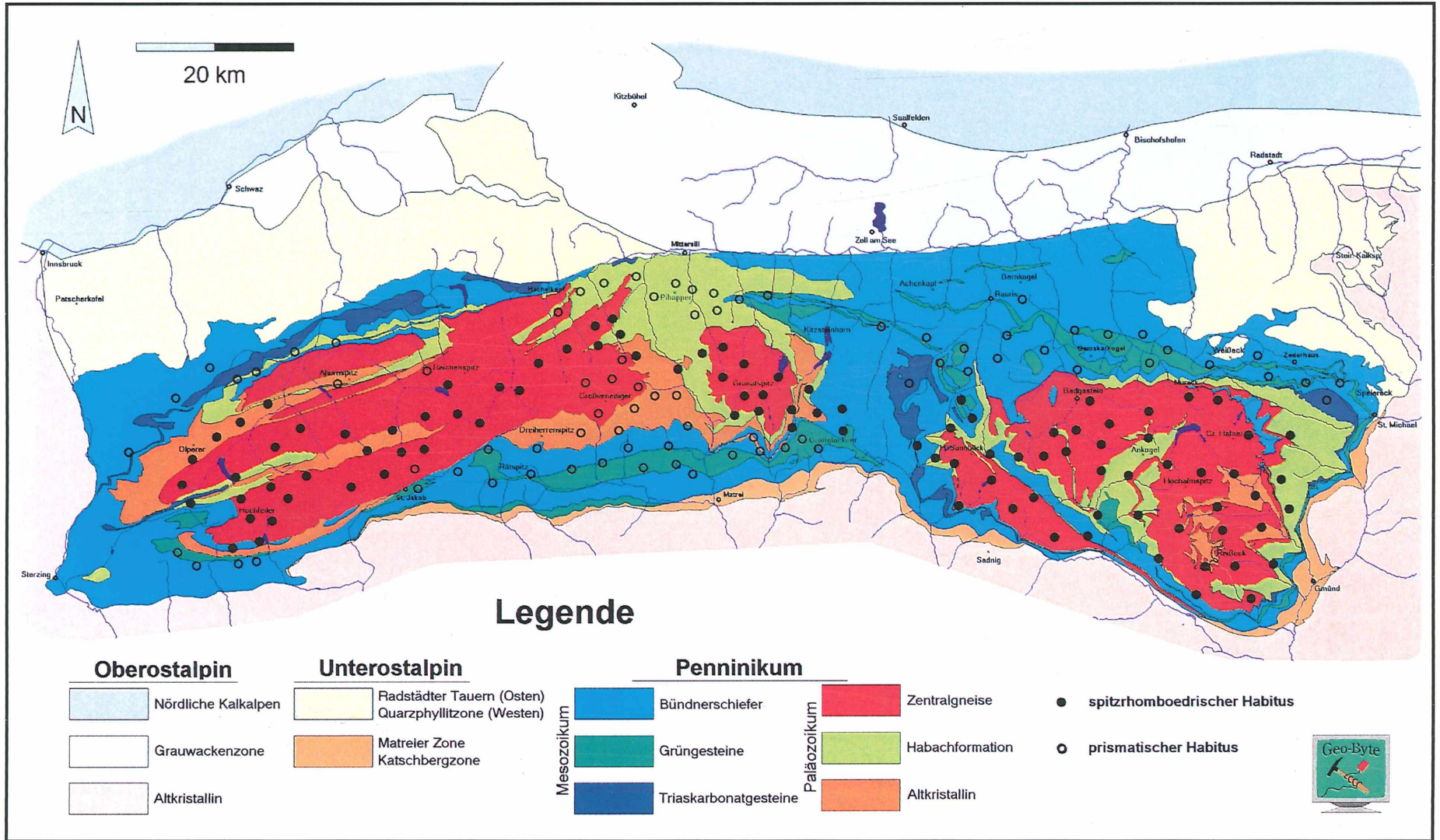
Abb. 3: Geologische Karte des Tauernfensters (vereinfacht); dunkle Kreise: Fundstellen von Kristallen mit spitzrhomboedrischem Habitus, helle Kreise: Kristalle mit prismatischem Habitus
