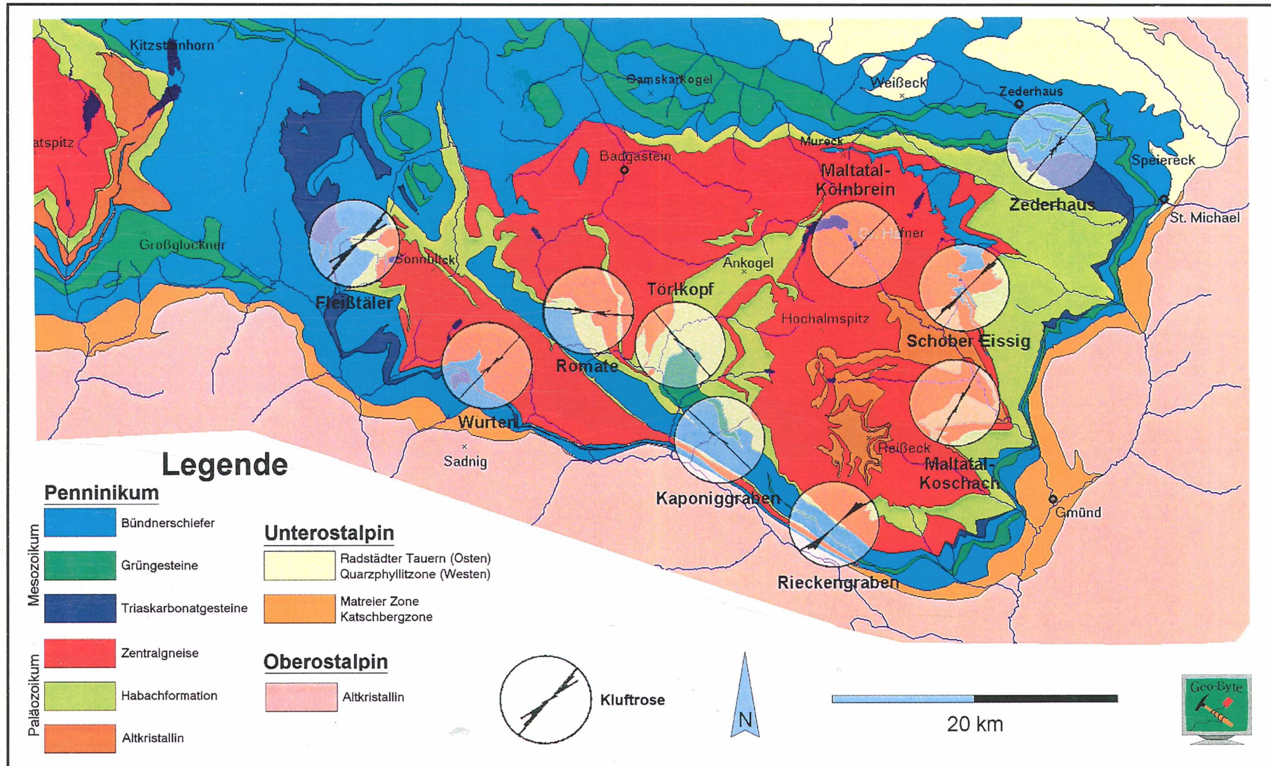
Abb. 2: Karte der Verteilung der Kluffrichtungen
