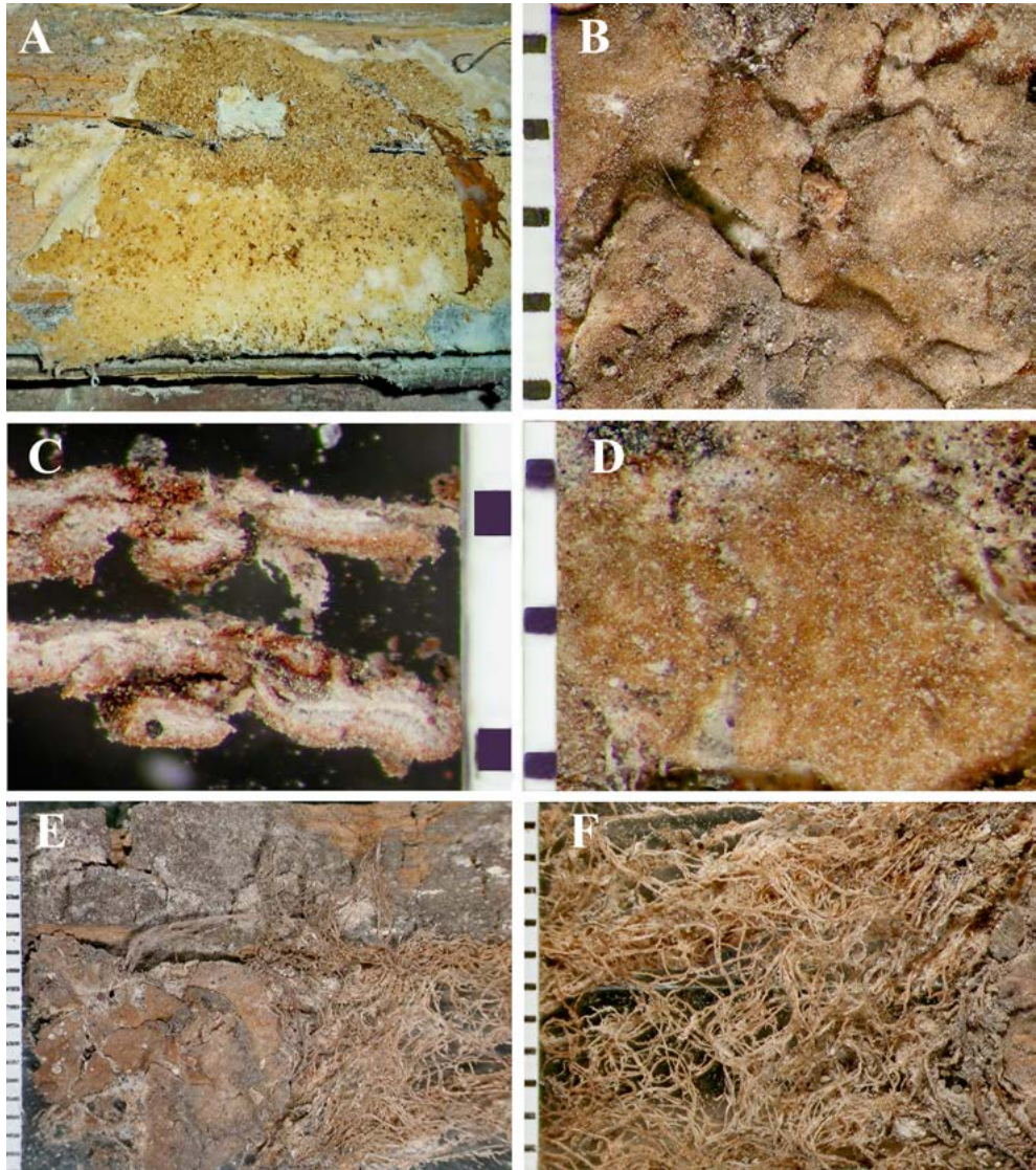
Abb. 2A-F: Fruchtkörper und Stränge von Coniophora prasinoides an Nadelholz des Fußboden-Aufbaus. A) frischer Fruchtkörper mit dünnem Rand auslaufend (vor Ort); B-F: Exsikkate; B) warziger Fruchtkörper im Detail (getrocknet, z. T. mit feiner Asche bedeckt); C) zwei Querschnitte eines Fruchtkörpers; D) glatter Fruchtkörper-Teil im Detail; E) Fruchtkörper mit Strängen auslaufend; F) feine, weiße bis hellbraune Stränge; Bilder B-F: Stacking-Bilder; Maßstäbe mit Millimetereinteilung. Foto 2A: P. v. D. HEIDE; Fotos 2B-F: T. HUCKFELDT
