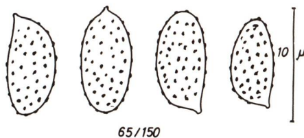
Abb. 2: Sporen von Dermocybe holoxantha . x 2000.
