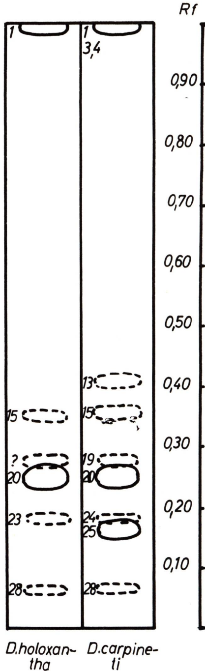
Abb. 3: Pigmentchromatogramme von Dermocybe holoxantha und carpineti (ined.). Die Numerierung bezieht sich auf eine noch unveröffentlichte Arbeit über die Pigmente in der Gattung Dermocybe . 1 : ?, 3 und 4 : Anthranol?, 13 : Cinnarubin?, 15 : Endocrocin, 19 : ?, rosa, 20 : Endocrocinglykosid?, 23 : Dermoluteinglykosid?, 24 : ?, rosa, 25 : ?, gelb, 28 : 5-Cl-Dermorubin?
