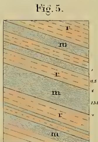
Bahnenschnitt bei Thiemendorf.
