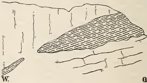
Zunge von Culmschiefer im devonischen Riffkalke des Mooskofels. Die mehrfach unterbrochene Fortsetzung ist nach W zu weithin am Abhange wahrnehmbar.
