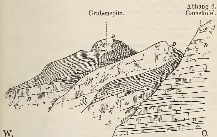
Das Ineingreifen von Culmschiefer (C) und Devonkalk (D) an der Grubenspitz.
