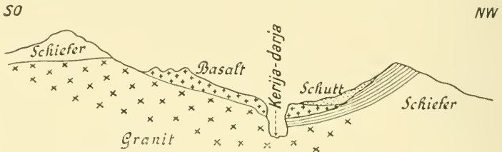
Querprofil des Tales des Kerija-darja nach ZUGMAYER.
