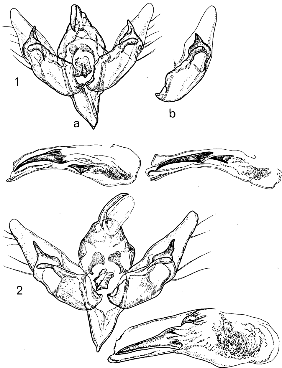
Abb. 4: ♂-Genitalarmaturen der Chersotis semna -Gruppe.
