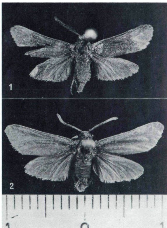
Abb. 1: ♂ von „ Ino kruegeri TURATI, 1930“ aus der „Typenserie“. Fundort: Scleidina, Cyrenaica, IV.; leg. Krueger. In Coll. Hartig (Bozen).
