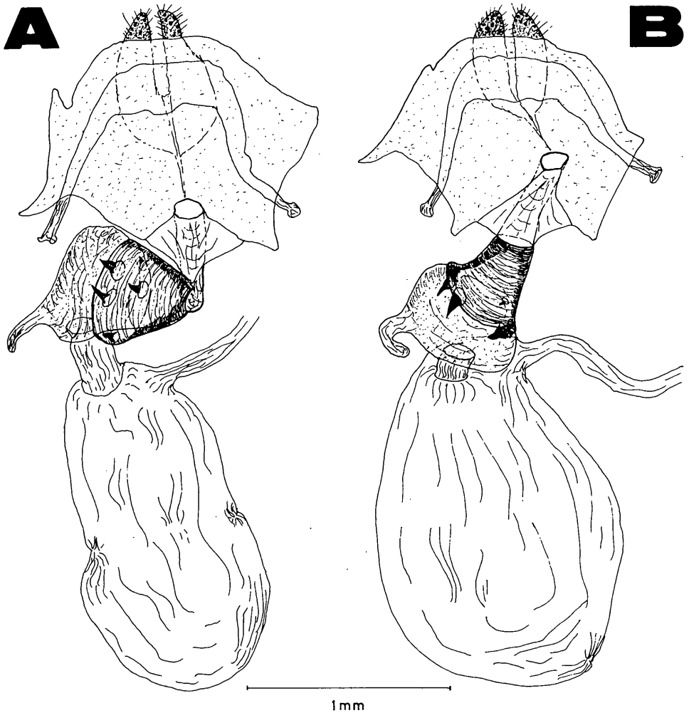
Abb.3: A – Genital ♀: „ Ino kruegeri TURATI, 1930“ aus der „Typenserie“. Fundort wie in Abb.1 und 2. Gen.Präp. Z 494 (Tarmann). In Coll. Hartig (Bozen). B – Genital ♀: Procris (Prav.) anatolica NAUFOCK, 1929. Fundort: Nahr el Kalb, Libanon, 3.-15.4.1968; leg. Ditgens. Gen.Präp. Z 393 (Tarmann). In Coll. Tarmann. Bei Abb.3 A befindet sich die Praebursa in natürlicher Lage. Sie steht im rechten Winkel (in ihrer Längsachse) zum Ductus bursae und Ductus intrabursalis. In Abb.3B ist sie etwas durch das Deckglas gequetscht und gedreht worden. In Präparaten mit Deckglas auf Objektträgern findet man meist diese Stellung vor. Sie entspricht nicht der natürlichen Lage der Praebursa!
