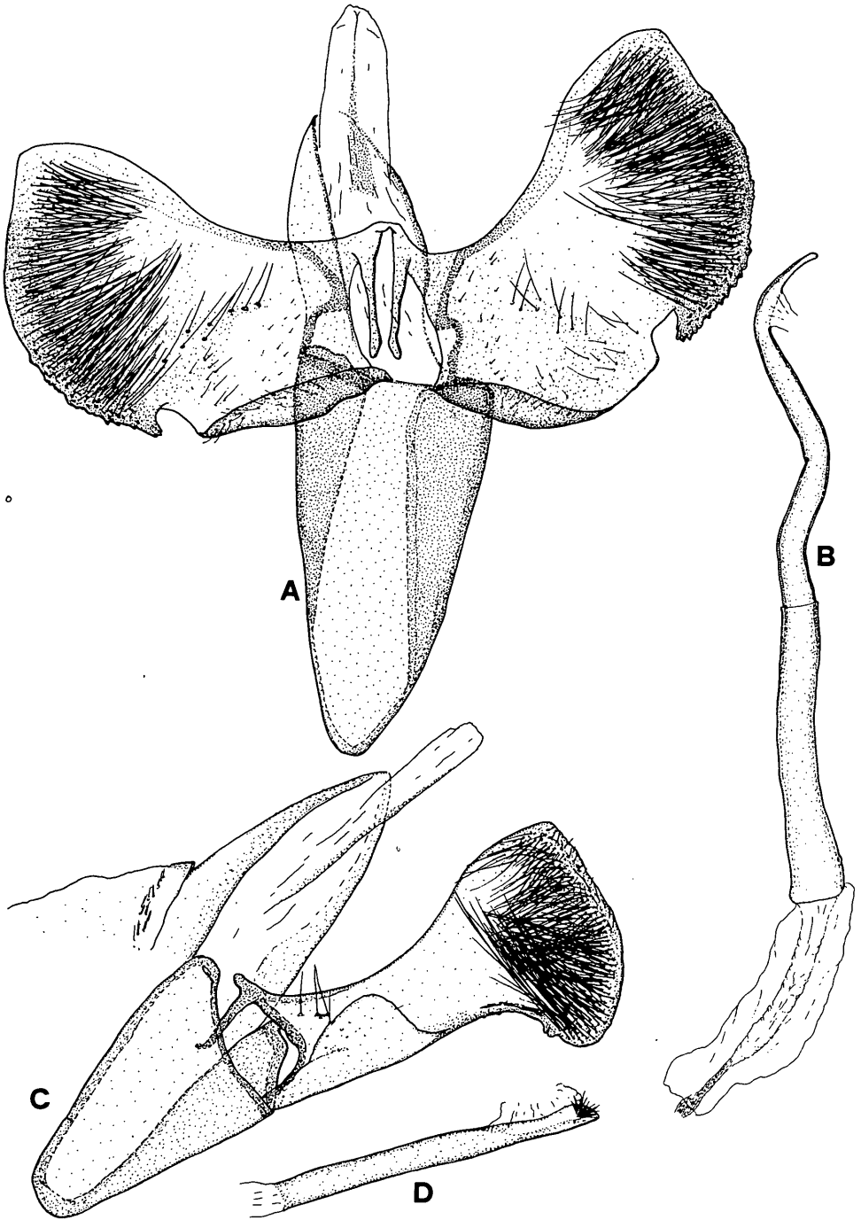
PLATE V. A - B: Aspilapteryx magna n.sp. A: Male genitalia; B: Aedoeagus. - C - D: A. seriata MEYR. C: Male genitalia; D: Aedoeagus.
