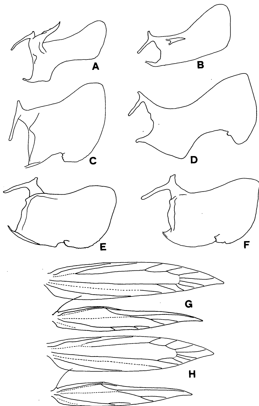
PLATE VII. A-F: valvae. A: A. limosella DUP.; B: A. inquinata n.sp., C: A. tringipennella Z.; D: A. seriata MEYR.; E: A. multipunctella CHRÉT.; F: A. magna n.sp. — G-H: wing venation. G: A. tringipennella Z.; H: A. limosella DUP.
