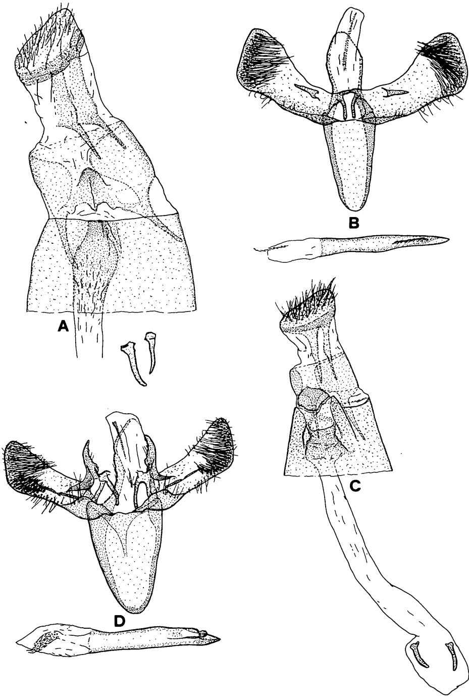
PLATE VI. A - B: Aspilapteryx inquinata n.sp. A: Female genitalia; B: Male genitalia. — C - D: Aspilapteryx limosella DUP. C: Female genitalia; D: Male genitalia.
