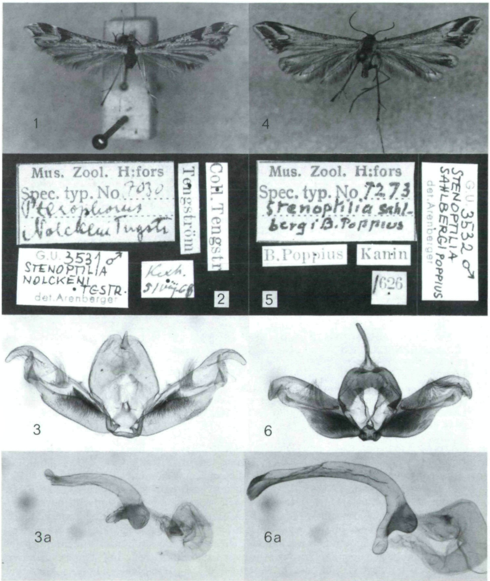
Abb.1: Stenoptilia nolckeni TENGSTRÖM, Paralectotypus; Abb.2: Etiketten des Lectotypus von St. nolckeni ; Abb.3: Männlicher Genitalapparat von St. nolckeni , Lectotypus; Abb.3a: dito, Aedoeagus; Abb.4: Paraplatyptilia sahlbergi POPPIUS, Paralectotypus; Abb.5: Etiketten des Lectotypus von P. sahlbergi ; Abb.6: Männlicher Genitalapparat von P. sahlbergi , Lectotypus; Abb.6a: dito, Aedoeagus.
