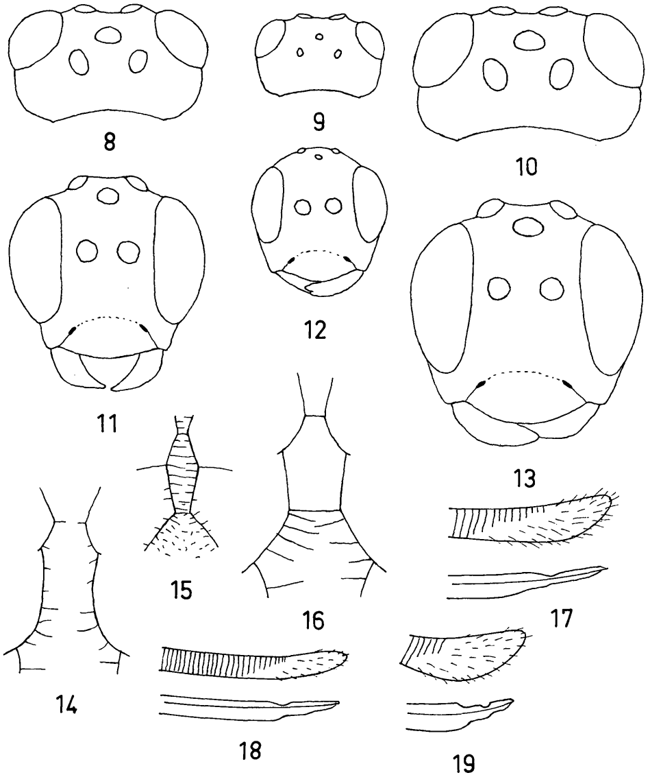
Abb. 8-10: Dorsalansicht des Kopfes. 8 - Leptoperilissus maroccanus (♀), 9 - L. microps (♀), 10 - L. persicus (♀). Abb. 11-13: Frontalansicht des Kopfes. 11 - L. maroccanus (♀), 12 - L. microps (♀), 13 - L. persicus (♀). Abb. 14-16: Bereich der Area superomedia. 14 - L. maroccanus (♀), 15 - L. microps (♀), 16 - L. persicus (♀). Abb. 17-19: Lateralansicht von Bohrer und Bohrerklappen. 17 - L. maroccanus (♀), 18 - L. microps (♀), 19 - L. persicus (♀).
