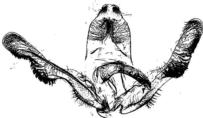
Abb. 1. Olethreutes concretanus , männliche Genitalien ( Phiaris stagnicolana , Lectotypus).
