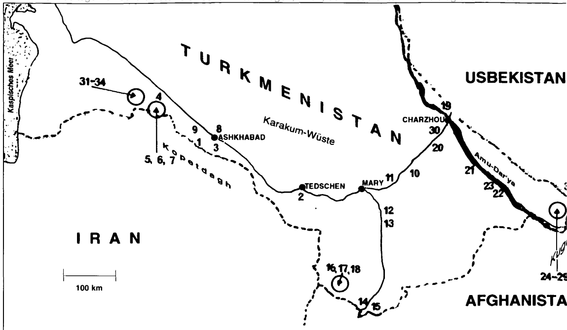
Abb. 1. Übersichtsskizze Turkmenistan. Die Nummern beziehen sich auf die im Text aufgelisteten Biotope.
