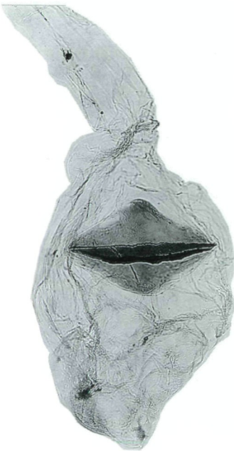
Abb. 9 - 12 Psamathocrita sp.: weibliche Genitalien (Signum doppelt vergrößert). (9-10) P. sp. , Ungarn (Gen.Präp. 3698 ZT); (11-12) P. sp. , Österreich (Gen.Präp. 3734 ZT).
