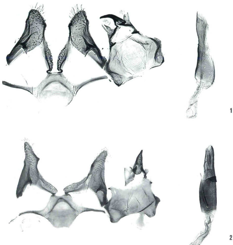
Abb. 1 - 2 Psamathocrita spp.: männliche Genitalien (aufgerollt). (1) P. dalmatinella sp.n., Kroatien (Gen.Präp. 00/900 PH); (2) P. osseella (STANTON), Schweden (Gen.Präp. 99/878 PH).
