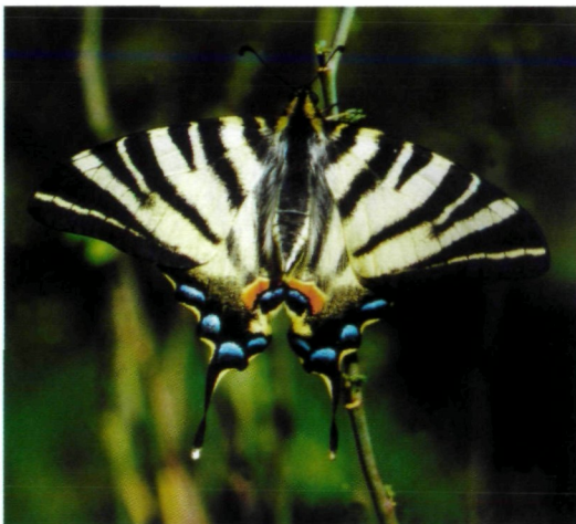
Abb. 2: Ipheclides podalirius tritt in Nordtirol nur sehr lokal an kleinklimatisch begünstigten Stellen auf.
