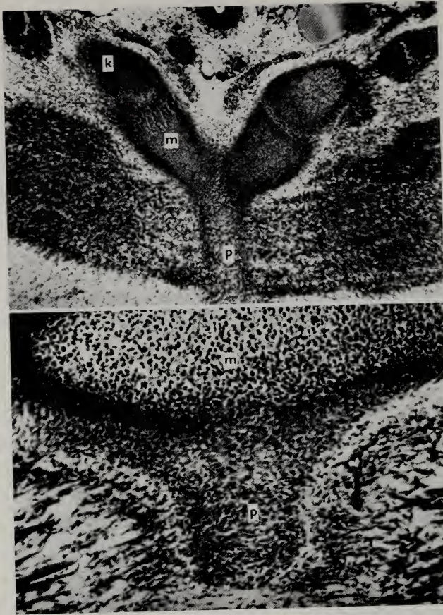
Abb. 2 (oben). Plecotus austriacus , Embryo 8 mm (75x). Querschnitt durch die paarige Anlage des Manubriums sterni (m) und die primäre unpaare Ventralanlage des Brustbeinkammes (p). Lateral sieht man die an das Sternum angeschlossenen Schlüsselbeine (k). — Abb. 3 (unten). Myotis myotis , Embryo 13 mm (200x). Querschnitt durch das Manubrium sterni (m) mit der primären Anlage (p) des Brustbeinkammes
