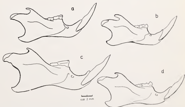
Abb. 6. Unterkiefer, Seitenansicht, Exemplare s. Abb. 2
