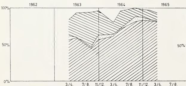
Abb. 3. Die Schwankungen in den Anteilen von M. arvalis , M. agrestis , Apodemus spec. und der übrigen Beutetiere in den Gewöllen der Waldohreule. — Neumünster
