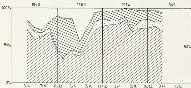
Abb. 2. Die Schwankungen in den Anteilen von M. arvalis , M. agrestis , Apodemus spec. und der übrigen Beutetiere in den Gewöllen der Waldohreule. — Husby
