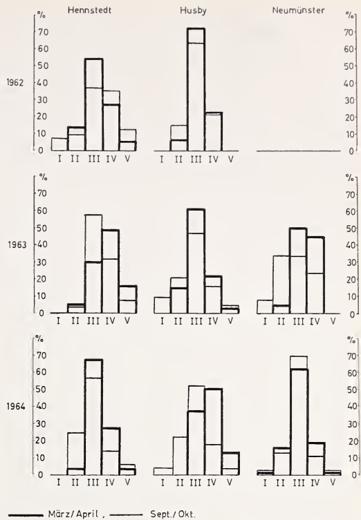
Abb. 8. Häufigkeitsverteilungen der Unterkieferlängen von M. arvalis aus Hennstedt, Husby und Neumünster. Übereinander projiziert sind jeweils die Frühjahrs- und Herbstaufsammlungen eines Jahres
