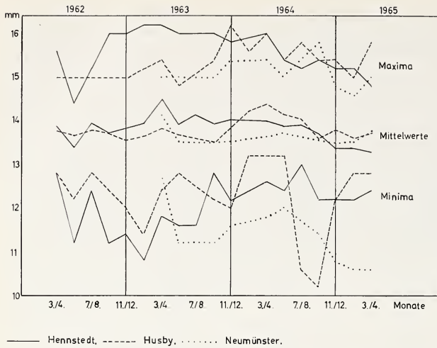
Abb. 4. Schwankungen der Mittel- und Extremwerte der Unterkieferlängen von Microtus arvalis in Hennstedt, Husby und Neumünster
