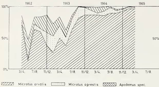
Abb. 1. Die Schwankungen in den Anteilen von Microtus arvalis , Microtus agrestis , Apodemus spec. und der übrigen Beutetiere in den Gewöllen der Waldohreule. — Hennstedt
