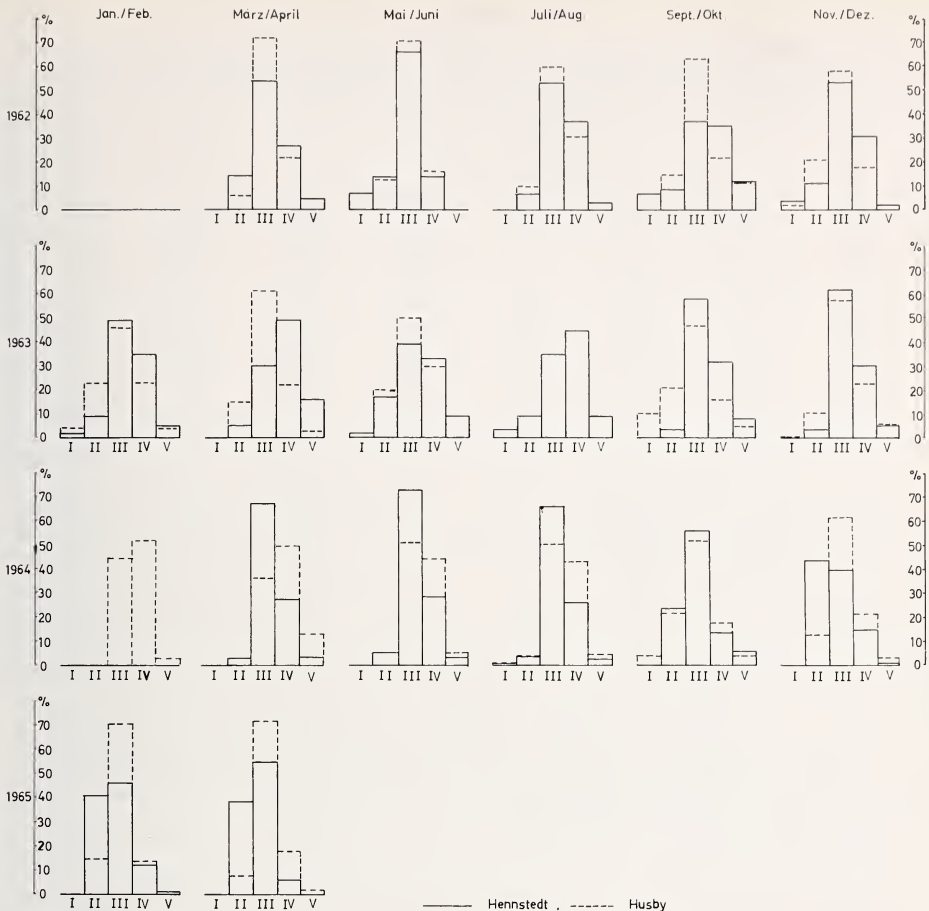
Abb. 5. Häufigkeitsverteilung der Unterkiefer-Längen von M. arvalis in zweimonatigen Intervallen aus Hennstedt und Husby
