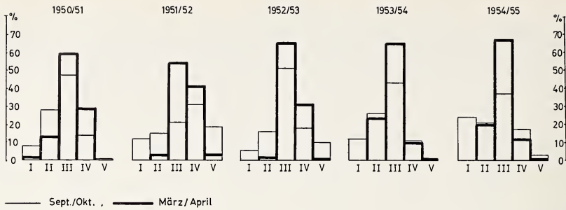
Abb. 7. Häufigkeitsverteilungen der Unterkiefer-Längen von M. arvalis aus Brandenburg (gezeichnet nach Daten aus ZIMMERMANN 1955)
