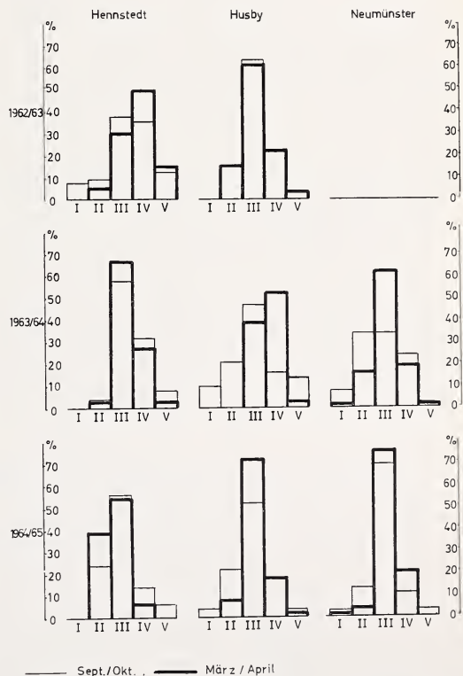
Abb. 6. Häufigkeitsverteilungen der Unterkieferlängen von M. arvalis aus Hennstedt, Husby und Neumünster. Übereinander projiziert sind jeweils die Vor- und Nachwinteraufsammlungen.
