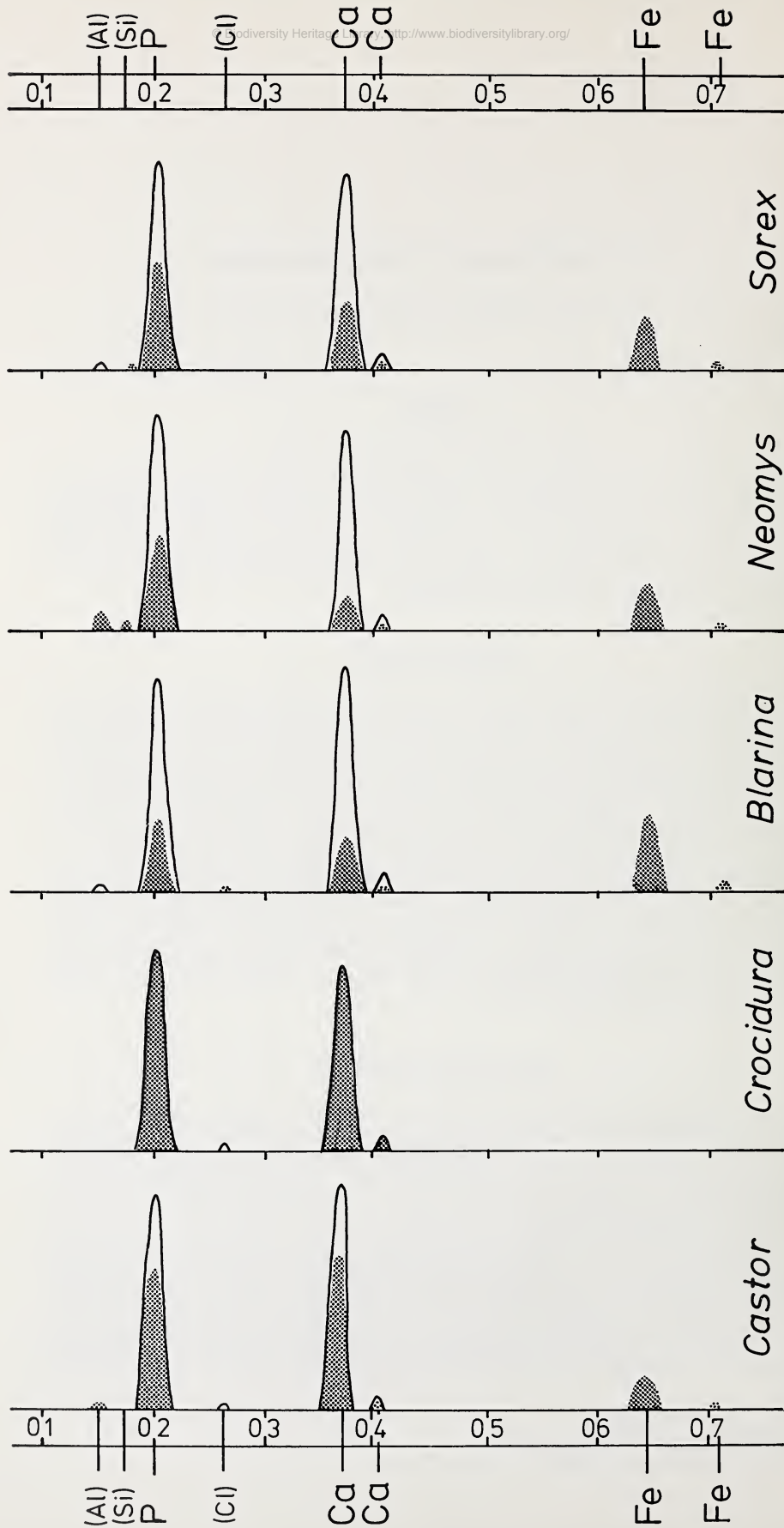
Abb. 1. Vergleich von äußerem, meist pigmentiertem (gerasterte Fläche) und innerem, stets unpigmentiertem Schmelz (unrandete Fläche) bei einigen Insectivoren und einem Rodentier ( Castor ) nach Messungen mit der Mikrosonde. Abszisse = Kanalnummern der X-Ray EDAX Mikrosonde; Ordinate = Anzahl der gemessenen counts. Für die Rotfärbung ist allein das Eisen verantwortlich.
