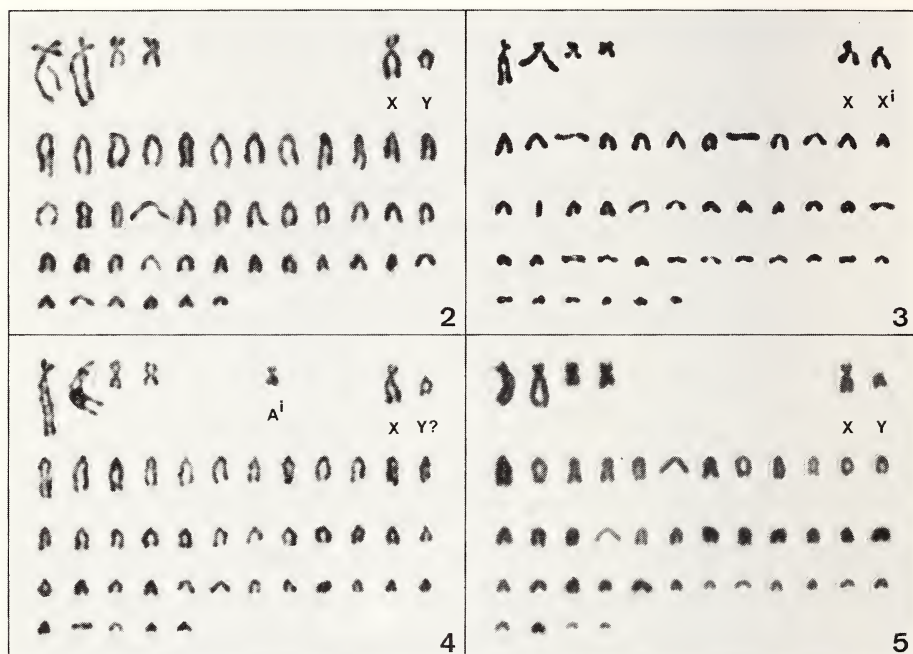
Fig. 2-5. Caryogrammes de P. multiplex . Fig. 2. ♂, 2N = 48 , NF = 54 , Sagno (Tessin) CH. Fig. 3. ♀, 2N = 48 , XX' , région de Briançon (Hautes-Alpes) F. Fig. 4. ♂, 2N = 48 , A' , Col de la Cayolle (Basses-Alpes) F. Fig. 5. ♂, 2N = 46 , NF = 52 , Fivizzano (Toscana) I
