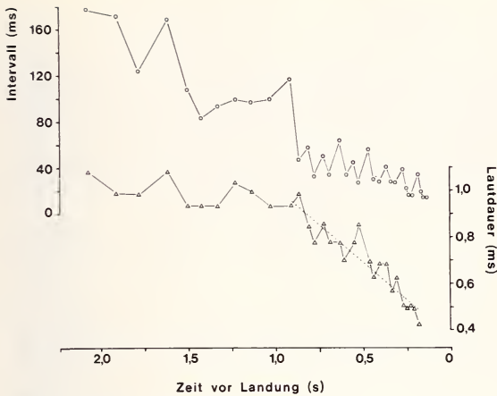
Abb. 2. Intervallzeit (Kreise, linke Ordinate) und Lautdauer (Dreiecke, rechte Ordinate) beim Landeanflug. Für die letzten 0,75 s wurde eine Annäherungsgerade für die zeitliche Änderung der Lautdauer errechnet (punktirierte Linie)
