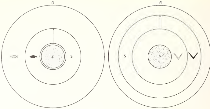
Abb. 4. Gesichtsfeld des Weißwalauges in 2,0 m Entfernung auf \frac{1}{25} verkleinert; P = für das Sehen leeres Gebiet des blinden Flecks; S = Ring scharfer Sicht, links im Wasser, rechts in Luft, G = Grenze des Sehfeldes unter einem Winkel von 80^\circ
