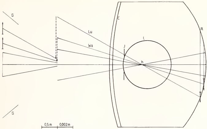
Abb. 3. Schema der Optik des Auges von Delphinapterus leucas . C = Cornea; L = Linse; R = Retina; I = Iris; h, h' = Hauptpunkte der Linse; P = Gebiet der Papille, blinder Fleck, linker Teil auf 1:25 verkleinert, rechts 10:1 vergrößert; wa = Verlauf eines Hauptstrahles im Medium Wasser; Lu = in Luft, Entfernung der Gegenstandsebene 2,0 m; G = Grenze des Sehfeldes unter einem Winkel von 80^\circ
