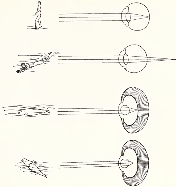
Abb. 1. Strahlengang im Auge des Menschen und des Weißwals in Luft und Wasser nach SLIJPER 1979)
