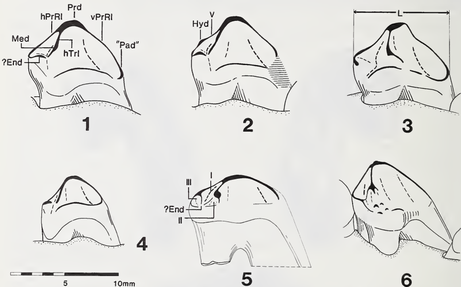
Abb. 3. Schematisierte Lingualansichten des P 3 sin. von Macaca sylvanus (rezent), Macaca sp. (Jungpleistozän, Österreich) und „ M. florentina “ (Altpleistozän, Italien); 1–3: M. sylvanus , männlich, UWPI 1324, NHMW 2614, NHMW 4408; 4: M. sylvanus , weiblich, NHMW 2616; 5: Macaca sp., männlich, Kugelsteinhöhle II, Steiermark; 6: „ M. florentina “, Strette, Val d’Arno, Altpleistozän, NHM Basel V.A.352, spiegelbildlich. Abkürzungen: Ci = Cingulum, End = Entoconid, iHl = innere Hauptleiste, hMeHl = hintere Metaconid-Hauptleiste, hPrRI = hintere Protoconid-Randleiste, hTrl = hintere Trigonidleiste, (= Protolophid), Hyd = Hypoconid, L = Meßstrecke der oberen Länge, Med = Metaconid, „Pad“ = Paraconid-Bezirk, Prd = Protoconid, Tag = Talonidgrube, Trg = Trigonidgrube, V = Vallis externus, Außental (= Hypoflexid), vEnRI = vordere Entoconid-Randleiste, vPrRI = vordere Protoconid-Randleiste; I, II, III = Teilgruben der Talonidgrube
