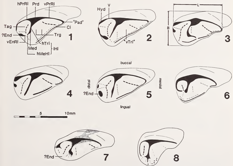
Abb. 4. Schematisierte Occlusalansichten des P_3 sin. von männlichen M. sylvanus (rezent), Macaca sp. (Jungpleistozän, Österreich) und „ M. florentina “ (Altpleistozän, Italien). 1–6: M. sylvanus , rezent. 1: UWPI 1324; 2: NHMW 2614; 3: NHMW 4408; 4: IPDW Nr. 4; 5: NHMW 2614 spiegelbildlich; 6: NHMW 32990; 7: Macaca sp., Kugelsteinhöhle II, Steiermark, Jungpleistozän; 8: „ M. florentina “, Strette, Val d'Arno, Altpleistozän, NHM Basel A.V.352, spiegelbildlich. (Abkürzungen siehe Abb. 3)
