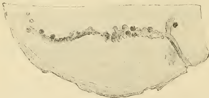
Fig. 1. Querschnitt des Frassganges von Sc. mikado in Acer pictum .
