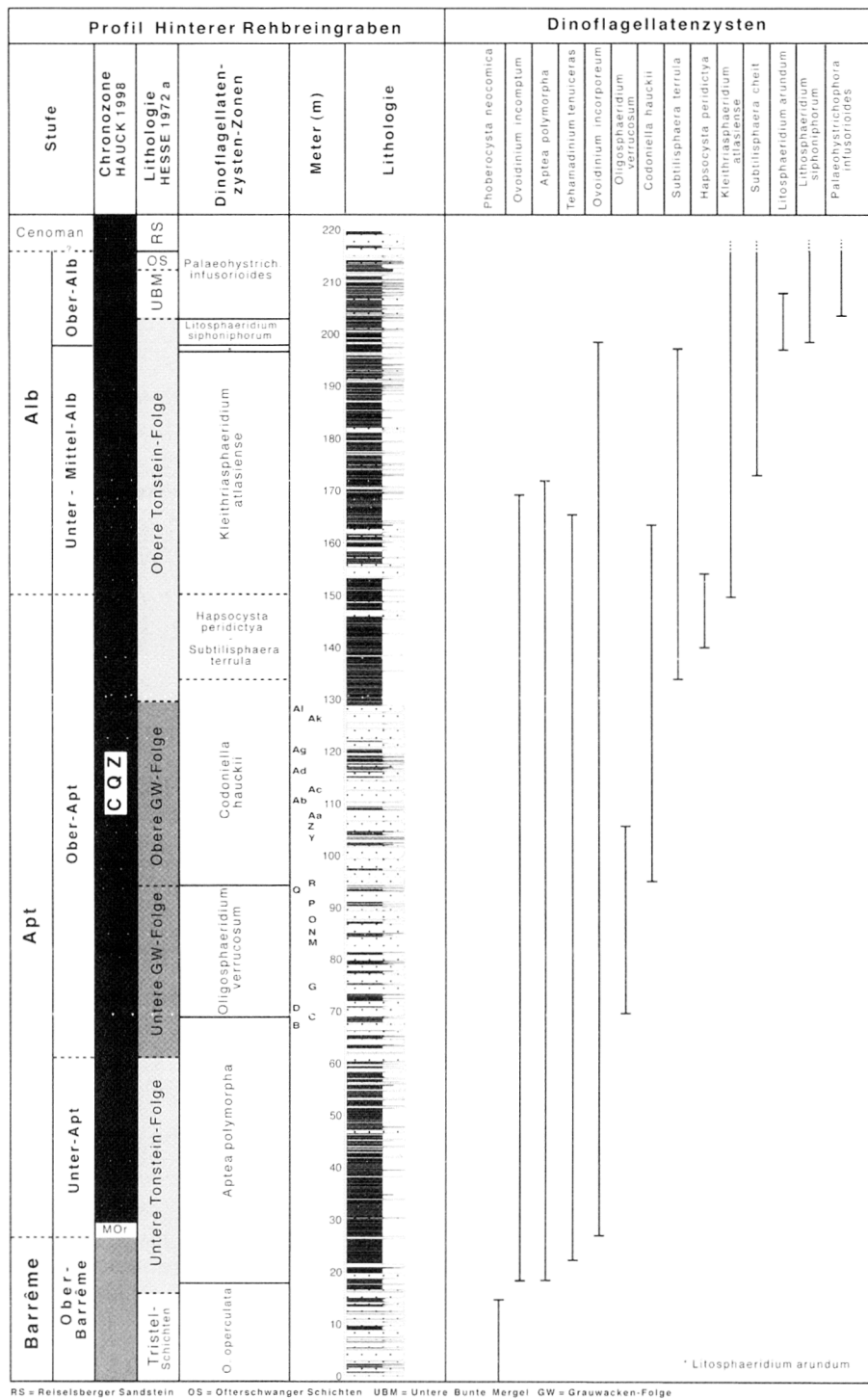
Abb. 3: Übersicht über das Gesamtprofil Hinterer Rehbrengraben (REB) mit stratigraphisch wichtigen Dinoflagellatenzysten nach KIRSCH (im Druck). Die Buchstaben in der Spalte Lithologie bezeichnen die Abfolge der Hartbänke im Bereich der Grauwacken-Folge (nach Hesse 1972a: P32).
