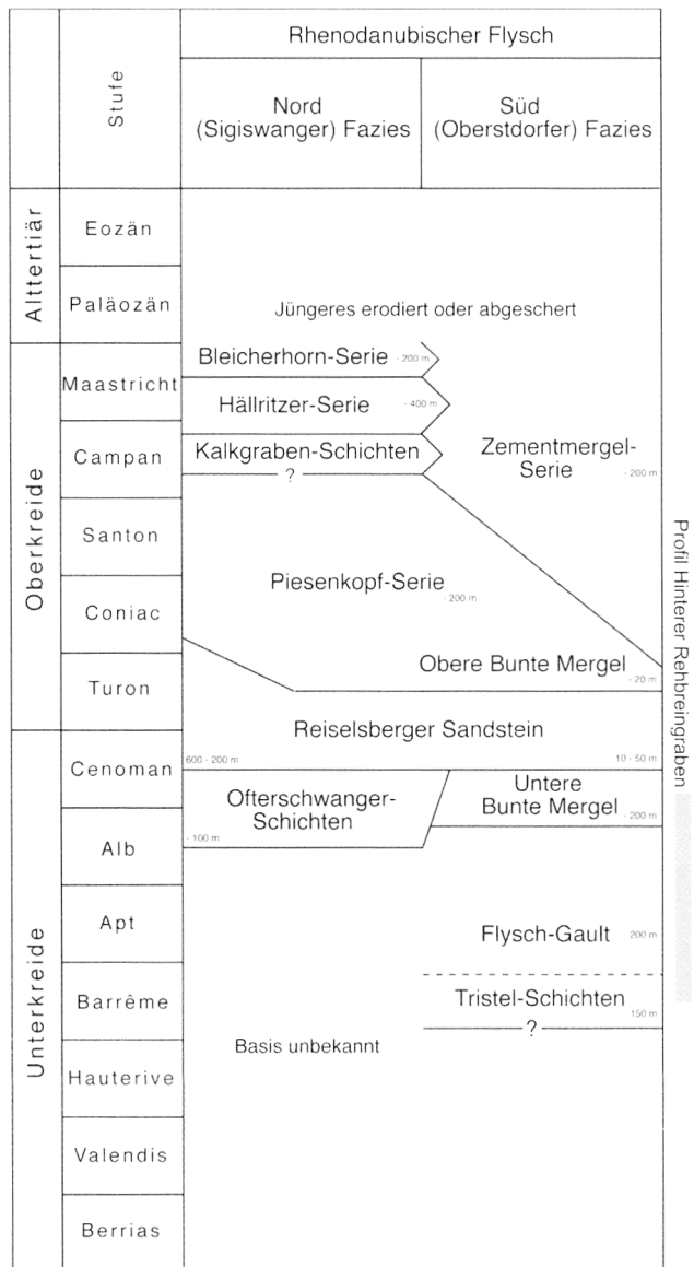
Abb. 2: Schichtenfolge der Rhenodanubischen Flysch-Zone (Oberbayern); aus KIRSCH (2000), modifiziert nach PFLAUMANN (1964: Abb. 3, 1968) und HESSE (1982, 1991: Abb. 2). Altersangaben aus HESSE (1991: 22 ff.) und KIRSCH (im Druck) sowie eigenen Angaben (siehe im Text).
