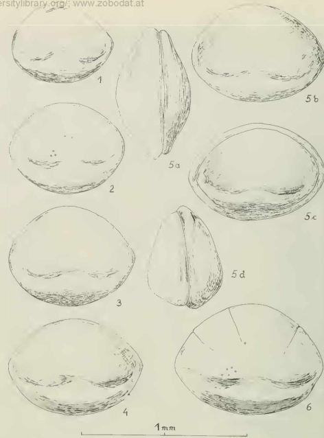
Abb. 5: Hermiella bagnii n. sp. aus Rhät-Mergel aus Bohrungen im südwestlichen Teil des Exmouth-Plateaus vor der NW-Küste Australiens. Fig. 1: linke larvale Klappe; Bohrung Eendracht-1, 2415-2425 m Bohrtiefe. Fig. 2: linke larvale Klappe; Bohrung Vinck-1, 2700-2710 m Bohrtiefe. Fig. 3: linke adulte Klappe mit besonders hohem Dorsalrand; Fundort wie Fig. 2. Fig. 4: Gehäuse von links, adult, zweiseitig symmetrisch, oben und unten gleich hoch gewölbt; Bohrung Investigator-1, 3295-3310 m Bohrtiefe. Fig. 5: Holotypus; a: Gehäuse von oben, b: G von links, c: G von rechts, d: G von vorne; Fundort wie Fig. 2. Fig. 6: Gehäuse von links, überaltert, dorsal etwas flachgedrückt; Fundort wie Fig. 4.
