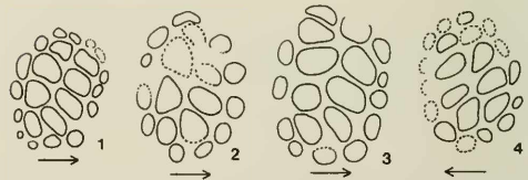
Abb. 2: Schließmuskelfelder von Hermiella ambo (LORD & MOORLEY, 1974). Germanischer Lias, Aubächle NW Asefingen, S-Württemberg, Süddeutschland; Material Tübingen Nr. 3762.
