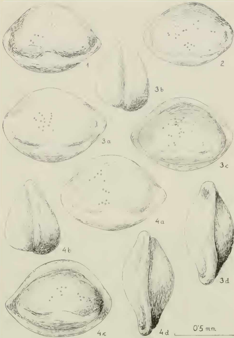
Abb. 4: Hermiella hermi n. sp. aus Rhät-Mergeln der Bohrung Investigator-1 im südlichen Teil des Exmouth-Plateau vor der NW-Küste Australiens; Fig. 1, 3, 4 aus 3295-3310 m Bohrtiefe, Fig. 2 aus 3320-3330 m. Fig. 1: Gehäuse von links mit distinkt zugespitztem Hinterende. Fig. 2: rechte Klappe. Fig. 3: Holotypus; 3a: G von links, 3b: G von vorne, 3c: G von rechts, 3d: G von oben. Fig. 4: Gehäuse mit besonders hohem Dorsalrand durch leichte Zusammendrückung; 4a: G von links, 4b: G von vorne, 4c: G von rechts, 4d: G von oben.
