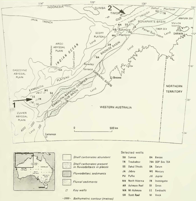
Abb. 1: Lage der Bohrungen mit den Hermiella beinhaltenden Rhät-Mergeln im südwestlichen Teil des Exmouth-Plateaus vor der nordwestlichen Küste Australiens (nach EXON et al. 1992: Abb. 6). Pfeil 1 zeigt auf die Bohrungen EE=Eendracht-1, IN= Investigator-1, VI= Vinck-1, SI= Sirius-1; von hier stammen die rhätischen Hermiellen des östlichen Formenkreises. Pfeil 2 zeigt auf den Fundort in Zentraltimor mit den liassischen Hermiellen des östlichen Formenkreises.
