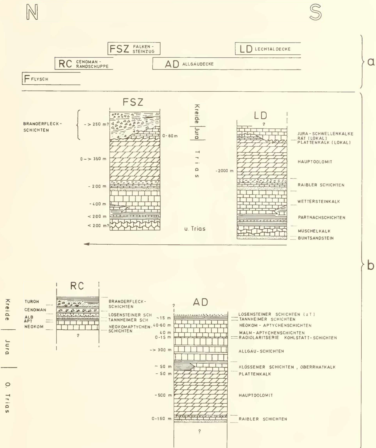
Abb. 2: Schematische Übersicht des Schichtbestandes verschiedener tektonischer Einheiten des Bajuvarikums (Ostallgäu und Tirol zwischen Lech und Iller).
