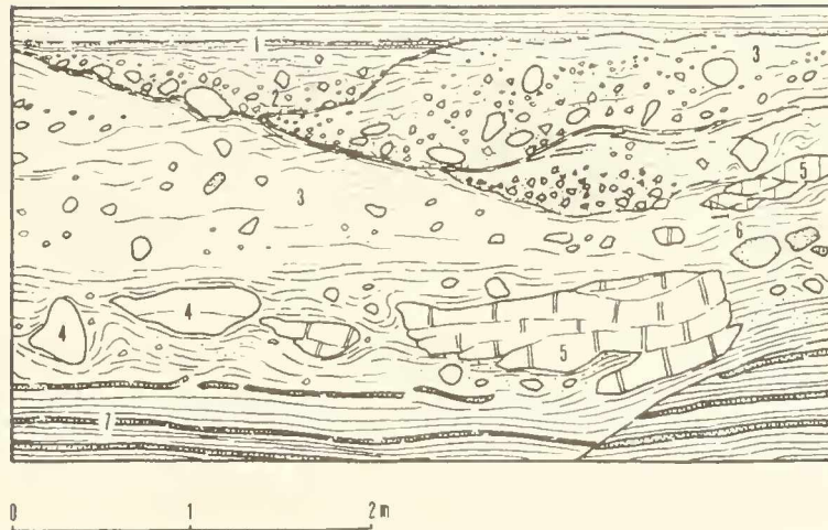
Abb. 7: Ausschnitt aus einem kleineren Olisthostrom der basalen Unteren Branderfleckschichten der Cenoman-Randschuppe (Vraconien).
