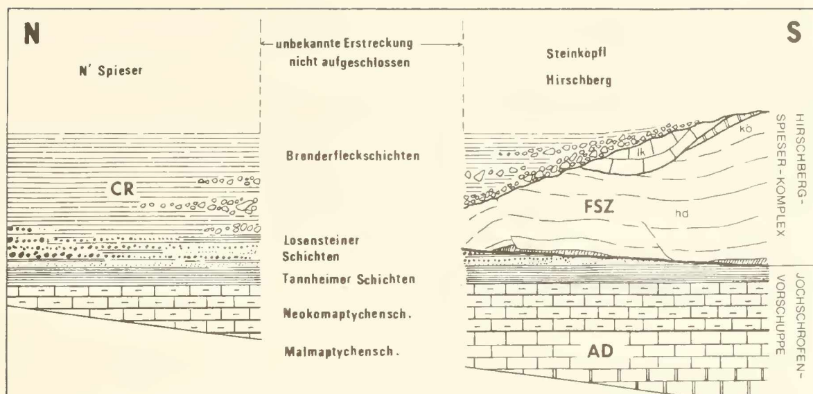
Abb. 13: Gegenüberstellung der Schichtfolgen und mögliche Beziehungen zwischen Cenoman-Bandschuppe (CR), Falkensteinzug (FSZ = Klippe der Lechtaldecken-Stirn) und Jochschrofen-Vorschuppe (zur Allgäu AD gehörig) zur Ablagerungszeit der Branderfleckschichten, nördlich Hindelang/Allgäu (ohne Maßstab, aus GAUPP 1977, ergänzt).
