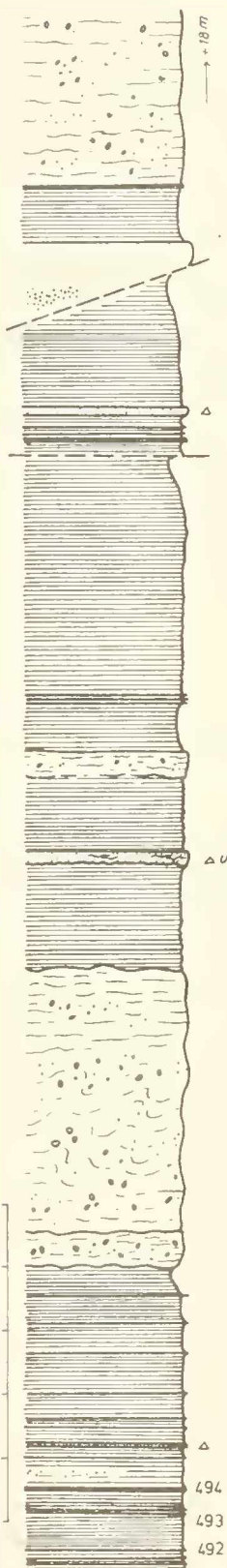
Abb. 5: Profilausschnitte von Losensteiner Schichten aus der Cenoman-Randschuppe nördlich Hindelang mit typischen Assoziationen der Lithofaziestypen.
