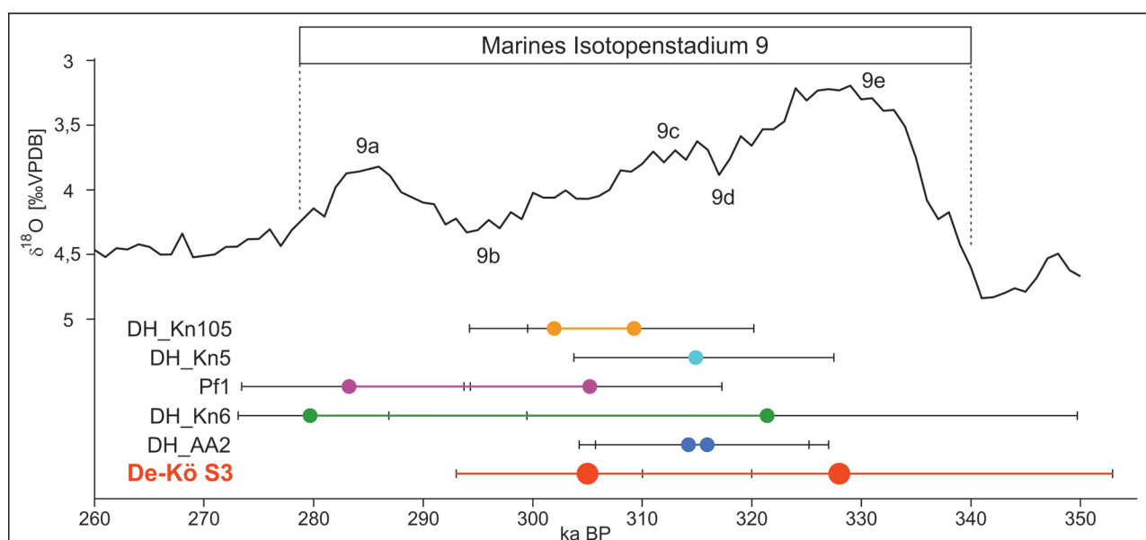
Abb. 11: ^{230}\text{Th}/\text{U} -Alter mit Fehlerbalken für den Stalagmiten De-Kö S 3 (rot) und für die noch hochaufgelöst zu bearbeitenden Stalagmiten. Im Vergleich der MIS 9-Abschnitt des \delta^{18}\text{O} -Profils für benthonische Foraminiferen nach Lisiecki & Raymo (2005).
