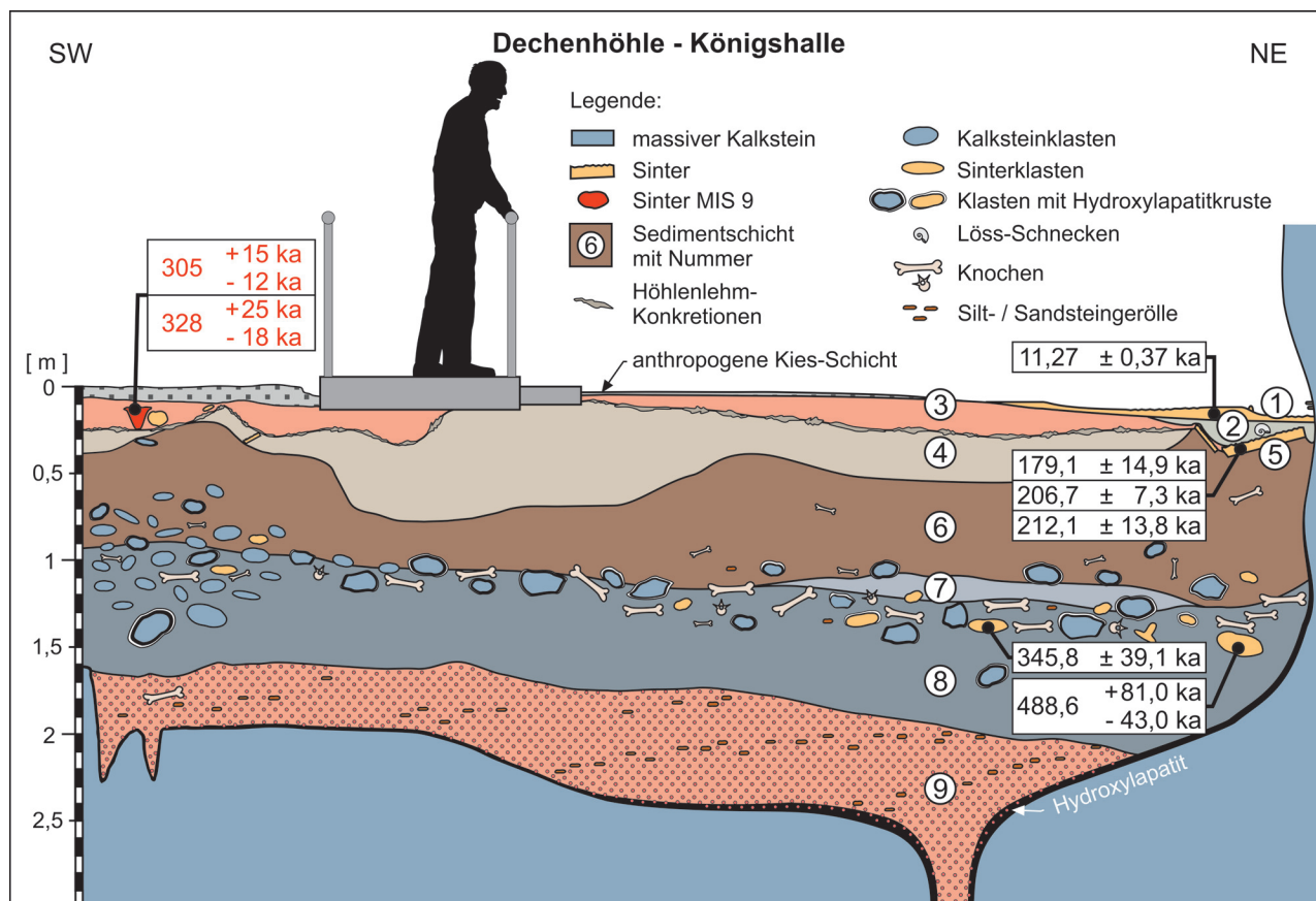
Abb. 4: Schemaprofil des Aufschlusses „Königshalle“; rot markiert: Holsteinbodensinter.
