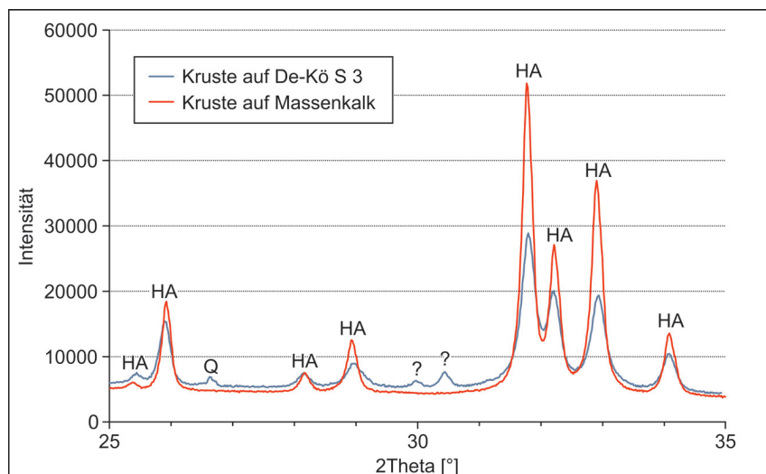
Abb. 10: Röntgendiffraktogramme für die Hydroxylapatitkruste mit Quarz auf dem Stalagmiten De-Kö S 3 und für eine reine Hydroxylapatitkruste vom NE-Abschnitt des Könighallenprofils (HA = Hydroxylapatit, Q = Quarz, ? = Crandallit/Woodhouseit).
