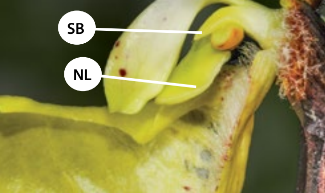
Abb. 6: Engstelle 1 - zwischen Steigborsten und Narbenlappen (NL). Zumindest nimmt die Sandbiene nun schon ein Licht am Ende des Tunnels wahr. Darüber steht auf beiden Seiten je ein Staubblatt (SB). Die Pollenmasse, die das Staubblatt produziert, ist klebrig.
