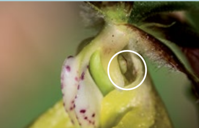
Abb. 7: Engstelle 2 - Das linke Schlupfloch als einer von zwei möglichen Fluchtwegen. Die Sandbiene kann nicht durch, ohne dabei auf ihrem Rücken Pollenschleim mitzunehmen.
